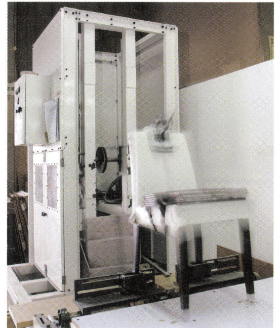
繰り返し衝撃試験を実施中のカトレア。
